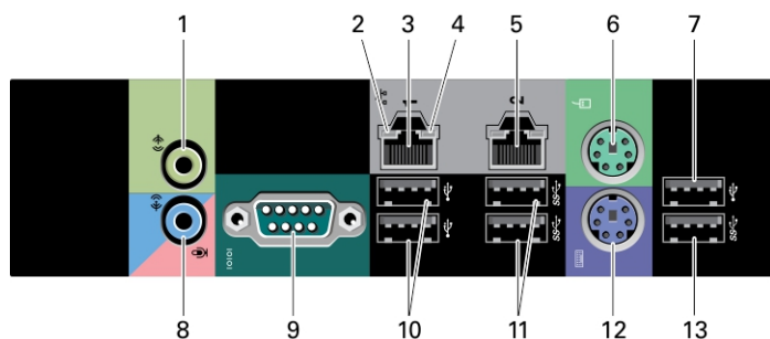
Figure 4. Vue du panneau arrière
